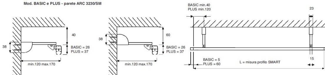
Mod. BASIC e PLUS - parete doppio ARC 3230
