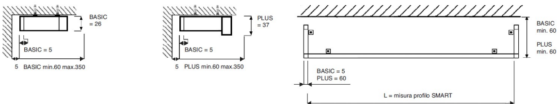
Mod. BASIC e PLUS - soffitto con angoli laterali
