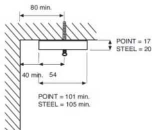
SOFFITTO CON SUPPORTO Art. 2740
