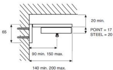
PARETE CON MENSOLE ARC Art. 3230/S
