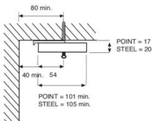
SOFFITTO CON SUPPORTO Art. 3239
