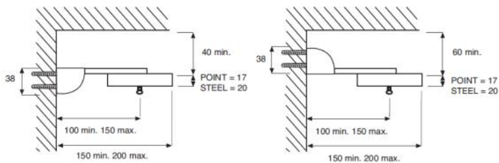
PARETE CON MENSOLE ARC Art. 3230/S
