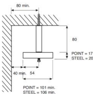
SOFFITTO CON SUPPORTO Art. 3216
