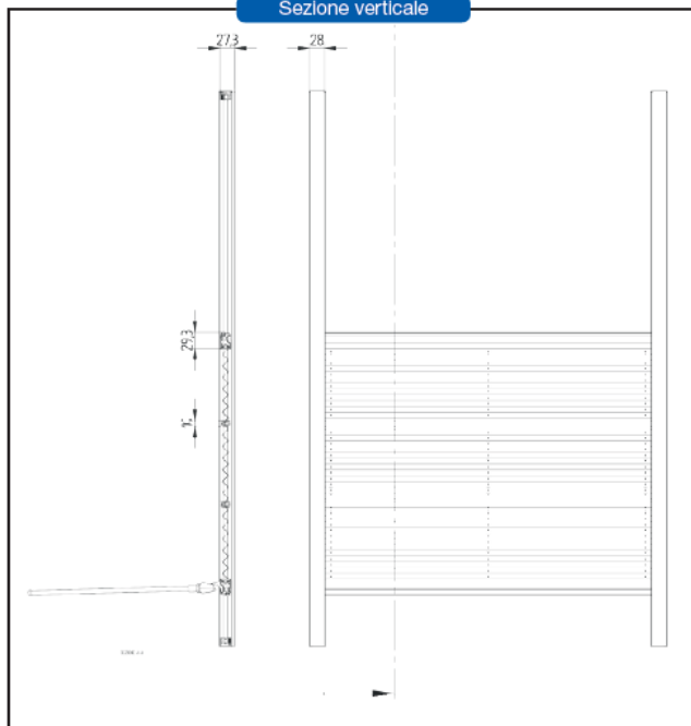
Sezione verticale
