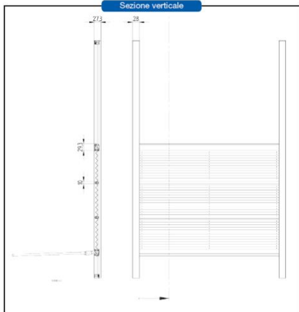
Sezione verticale
