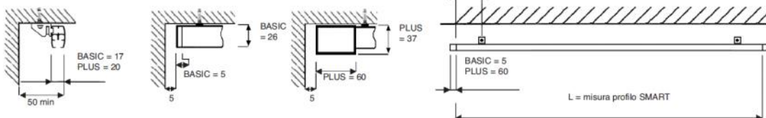
Mod. BASIC e PLUS - soffitto centinato
