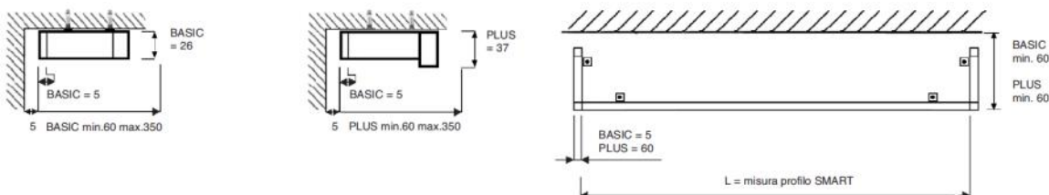
Mod. BASIC e PLUS - soffitto con angoli laterali
