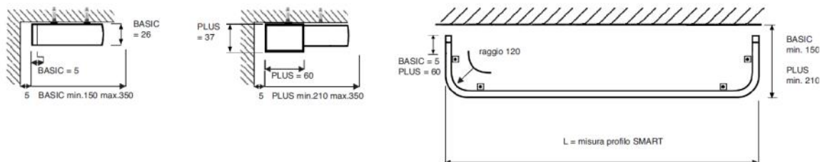
Mod. BASIC e PLUS - soffitto con angoli laterali
