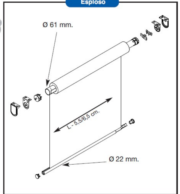
Esploso
