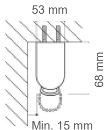
A soffitto Art. 8601K
