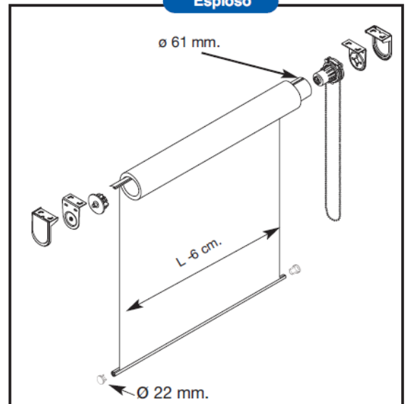
Esploso
