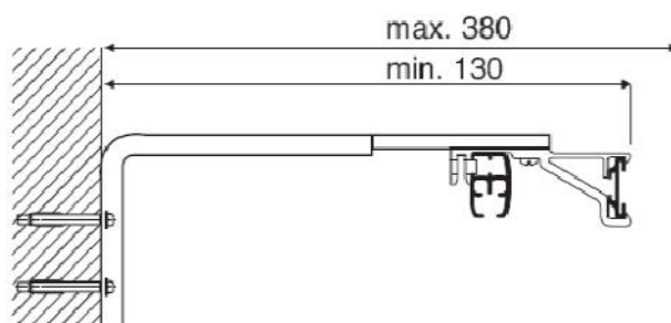
Art. 2721+2714+2725/10+2722
