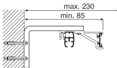
Art. 2721+2723+2725/20+2722
