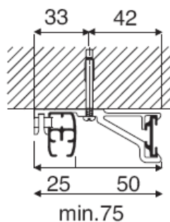
Art. 2722
