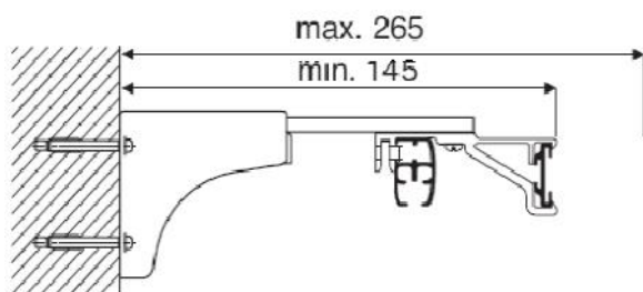
Art. 2713+2714+2722
